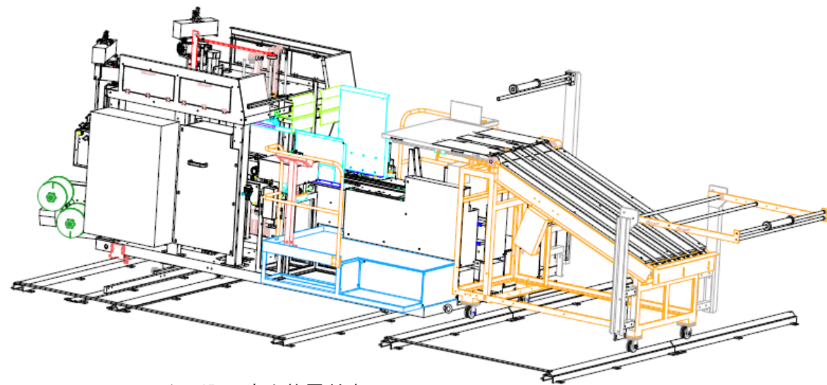
くい込み防止装置付き AA11-YTC90-KD型 (処理能力 MAX 16束/分) (図面は特別仕様です)
